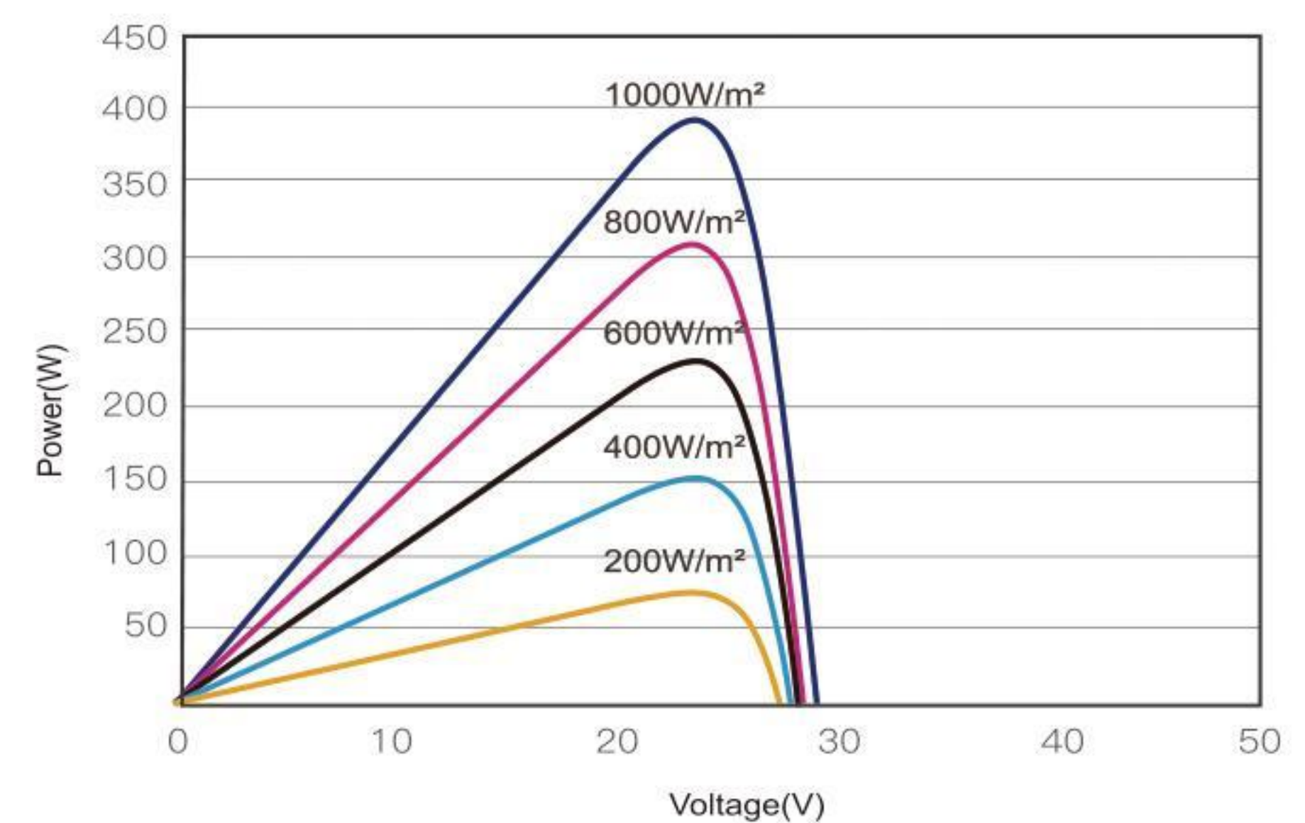
不同辐照度下电流电压曲线/功率电压曲线(395W)
